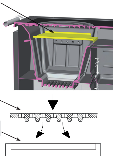
RAVNA REŠETKA IZ SIVE LITINE
